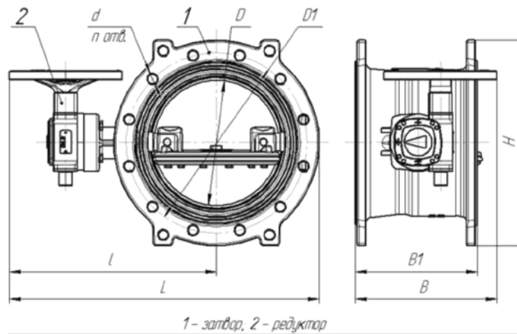
ГАБАРИТНЫЕ, УСТАНОВОЧНЫЕ, ПРИСОЕДИНИТЕЛЬНЫЕ РАЗМЕРЫ И МАССА, PN 10
