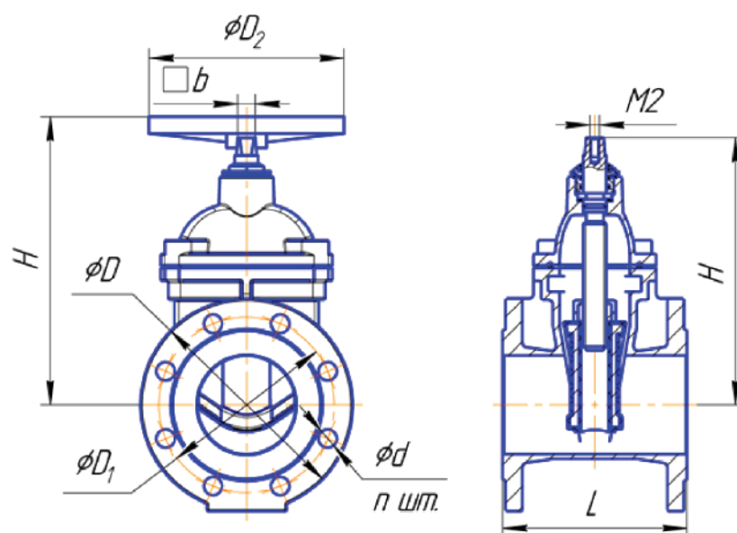
Габаритные, установочные, присоединительные размеры и вес задвижек со штурвалом
